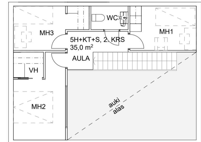
ASUNTOPOHJA, 2. KERROS 1:100
