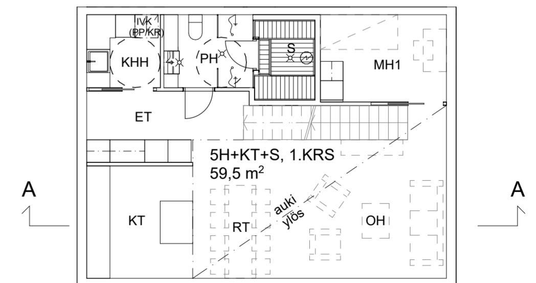
ASUNTOPOHJA, 1. KERROS 1:100
