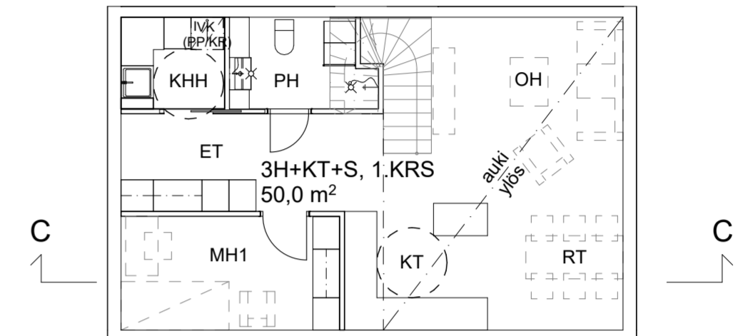
ASUNTOPOHJA, 1. KERROS 1:100
